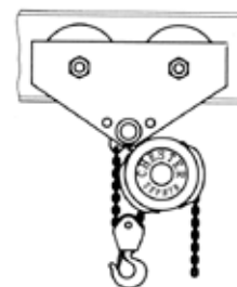
3 and 4 Ton (3 thru 10 Ton style)
